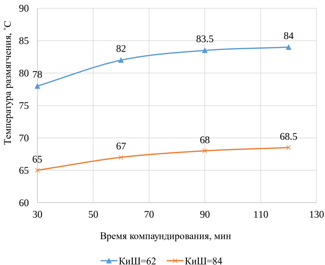
Рисунок 1 – График зависимости температуры размягчения от времени компаундирования.
