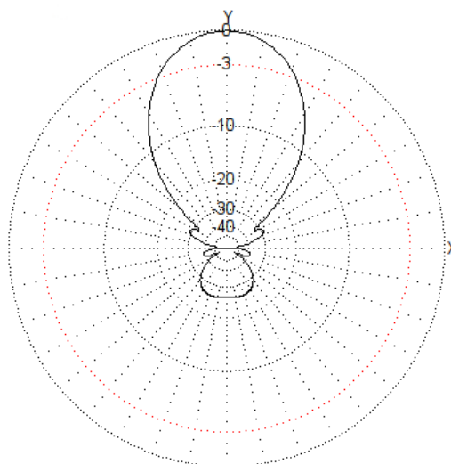
Рисунок 1: Диаграмма направленности
